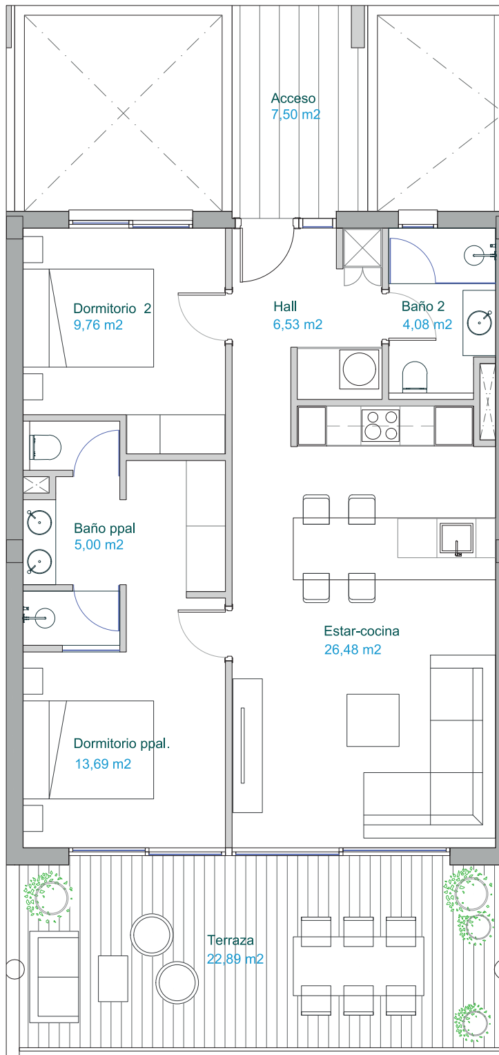
PLANTA. Escala_1/80
