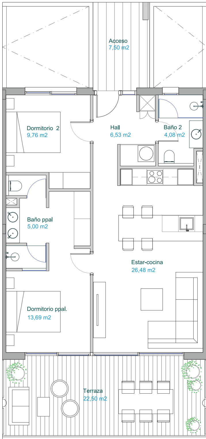
PLANTA. Escala_1/80
